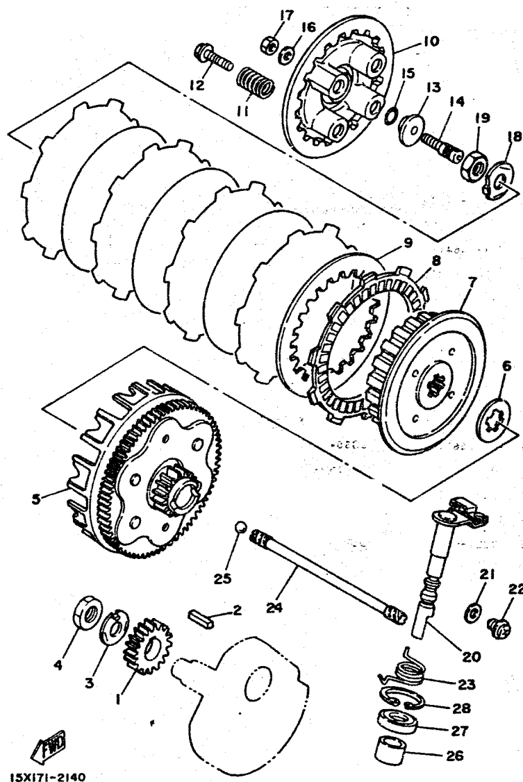
FIG. 14 CLUTCH
